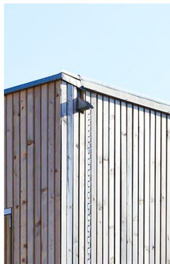
Trou d'évacuation des eaux avec protection
